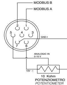
DETTAGLIO CONNESSIONI
